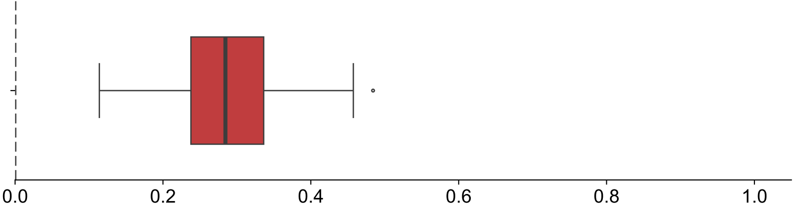
Steiner Subspace
